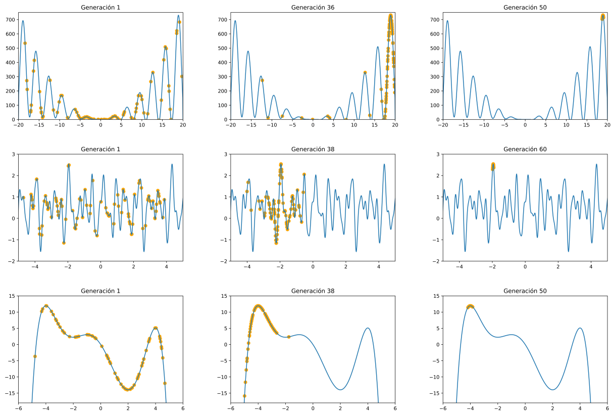
Figura 4.15: Exploración del espacio de búsqueda para diferentes generaciones. La línea azul representa los función de la cual buscamos el máximo. Los diferentes puntos amarillos representan a cada uno de los individuos.
