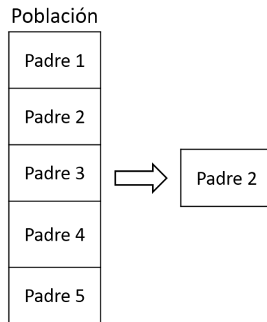
Figura 4.6: Representación de selección de aleatoria. Cada individuo tendrá la misma probabilidad de ser seleccionado.
