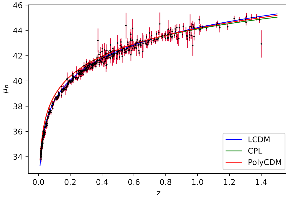
Figura 2.3: Datos de SNIa. Las líneas sólidas corresponde diferentes ajustes.
