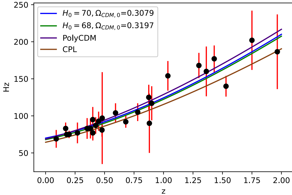
Figura 2.2: Datos de Hubble en función del corrimiento al rojo z para los cronómetros cósmicos. Las líneas sólidas corresponden a diferentes ajustes.
