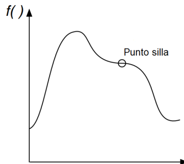
Figura 3.1: Representación de punto silla.
