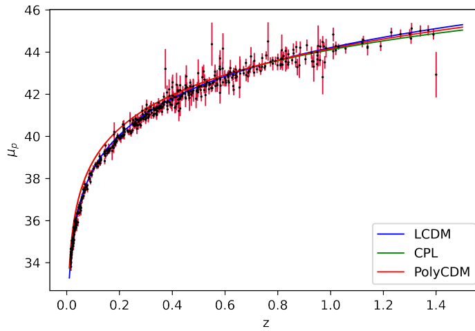
Figura 5.2: Datos de UnionSN. Este conjunto de datos representa la el módulo de distancia y el corrimiento al rojo para 580 supernovas.
