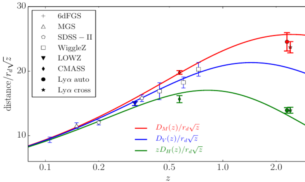
Figura 2.4: Datos de BAO a partir de las fuentes indicadas en la leyenda. El factor de escala \sqrt{z} se incluye para una mejor visualización de las barras de error. Las líneas sólidas se trazan utilizando los valores de mejor ajuste obtenidos por el satélite Planck [5]
