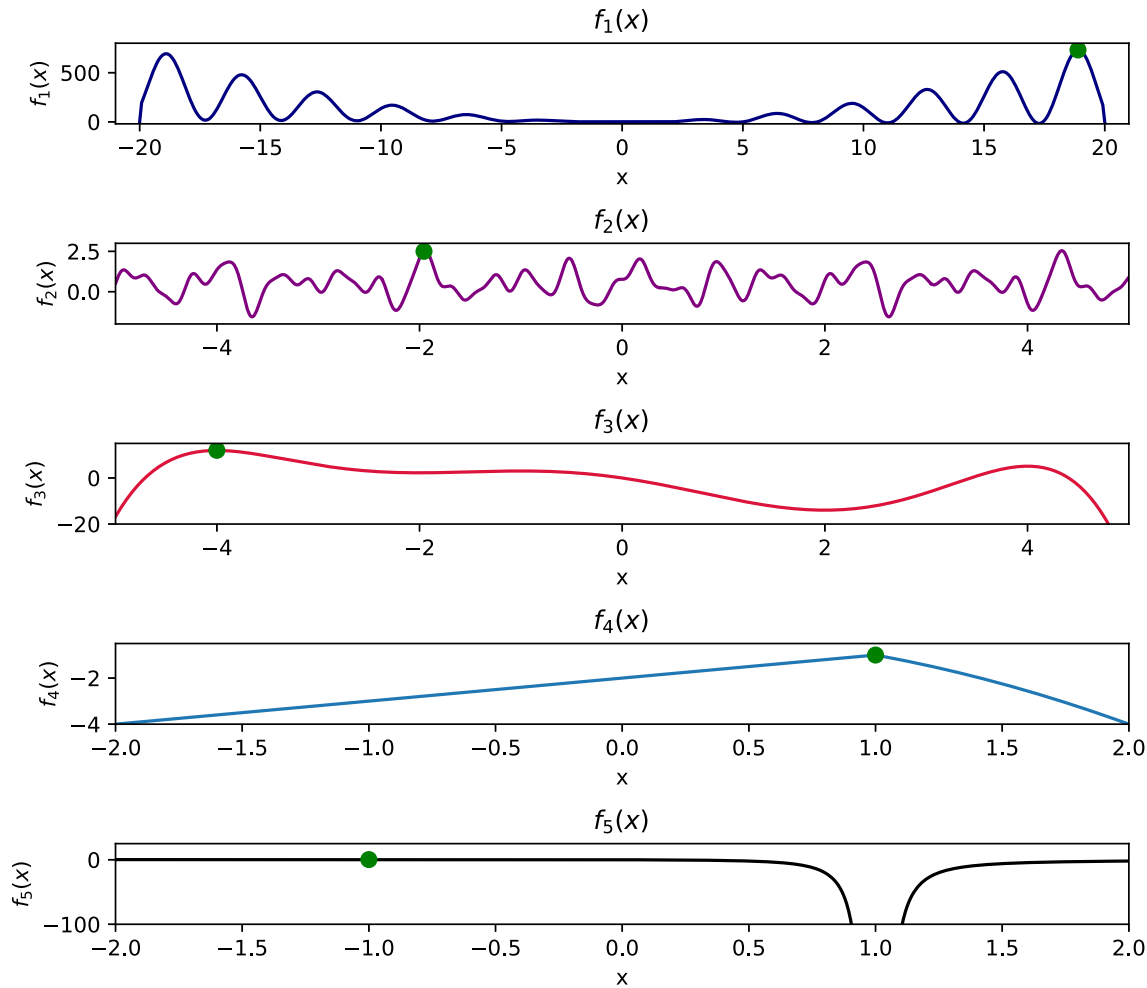
Figura 4.14: De arriba hacia abajo, gráficas de ecuaciones (4.2), (4.3), (4.4), (4.5) y (4.6) con sus mejores individuos en verde: 18.90, -1.95, -4.00, 1.00 y -1.00.
