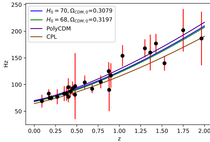
Figura 5.3: Se presentan los tres diferentes ajustes para cada modelo. Línea azul representa \Lambda CDM con valor fijo de H_0 = 70 , línea verde representa mismo modelo pero sin ningún valor fijo, por último línea morada representa el ajuste al modelo PolyCDM.
