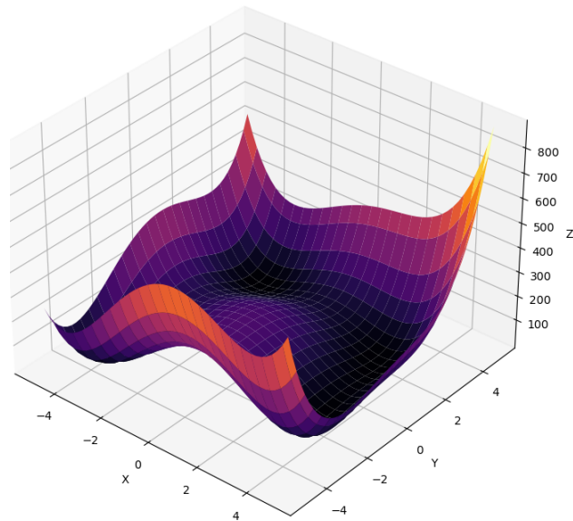
Figura 4.16: Función de Himmelblau
