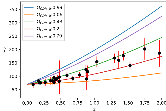
Figura 5.1: Ajuste del modelo 2.28 para diferentes valores aleatorios de \Omega_{\Lambda,0} , \Omega_{CDM,0} y un valor fijo de H_0 = 70 para conjunto de datos H(z) .
