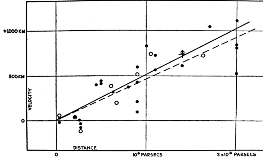
Figura 2.1: Gráfica original de Edwin Hubble de la relación entre el corrimiento al rojo (eje vertical) y la distancia (eje horizontal). Obsérvese que el eje vertical en realidad traza cz en lugar de z y que las unidades se escriben accidentalmente como km en lugar de km/s .
